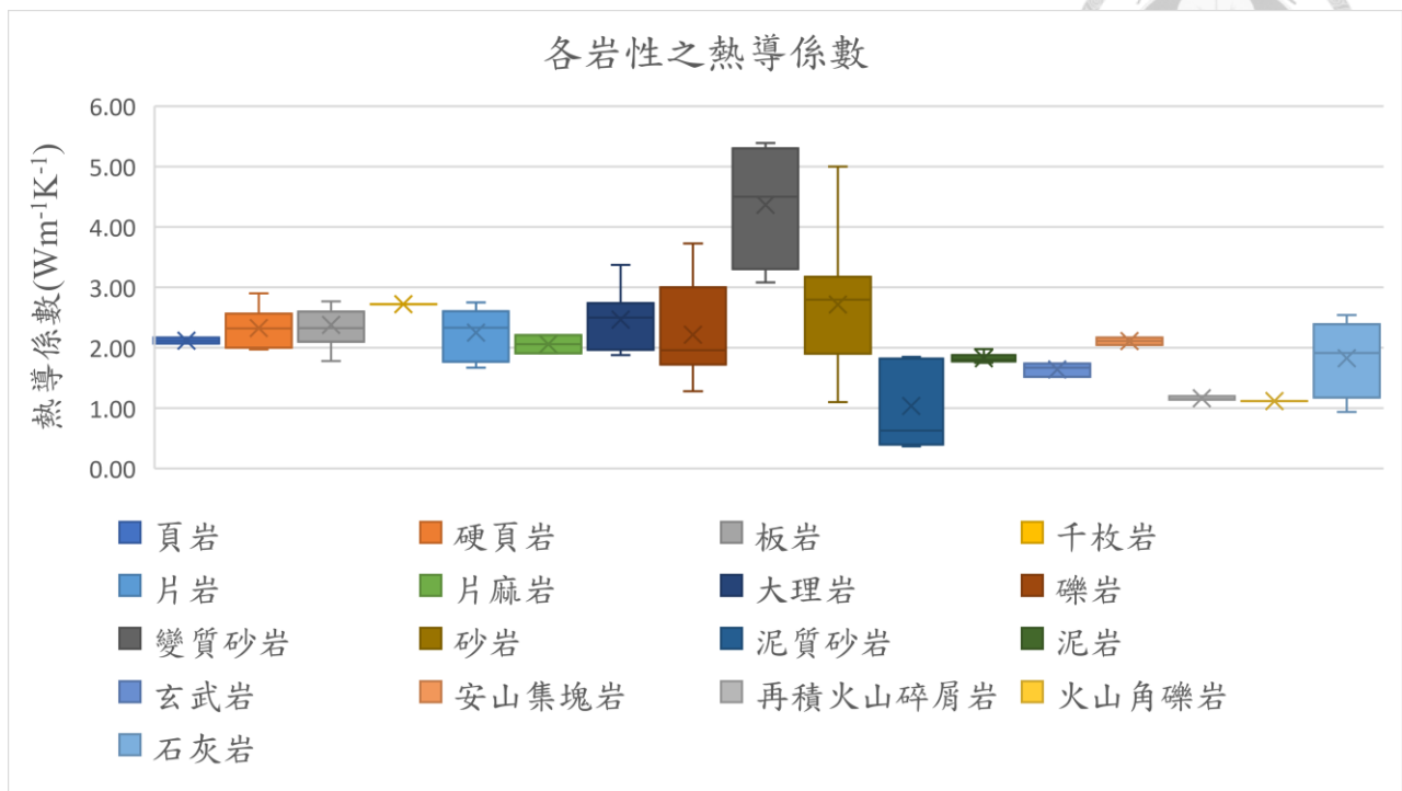
圖 3-5-1、各岩性之熱導係數盒鬚圖。X 表示該地質年代的平均值。圖中可看見臺灣各種岩性中，最大值出現在變質砂岩，最低值出現在泥質砂岩，熱導係數值範圍最大為砂岩 3.90 \text{ Wm}^{-1}\text{K}^{-1} ，扣除樣本數只有一個這類不具統計意義的岩性，範圍最小為再積火山碎屑岩 0.06 \text{ Wm}^{-1}\text{K}^{-1} 。
