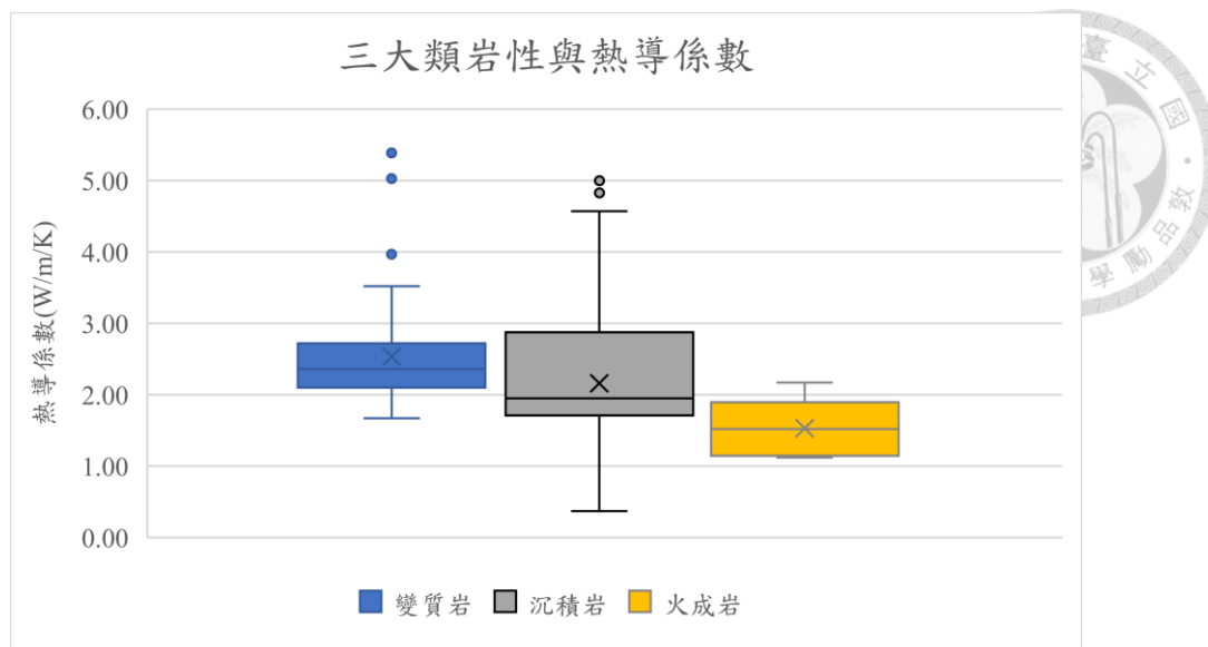
圖 4-2-3、三大類岩性與熱導係數盒鬚圖，圖上的點為該類岩性的極端值，極端值為距離第一、第三四分位數的距離超過盒子長度的 1.5 倍，完整解釋盒鬚圖可參考 Banks et al. (1998)。
